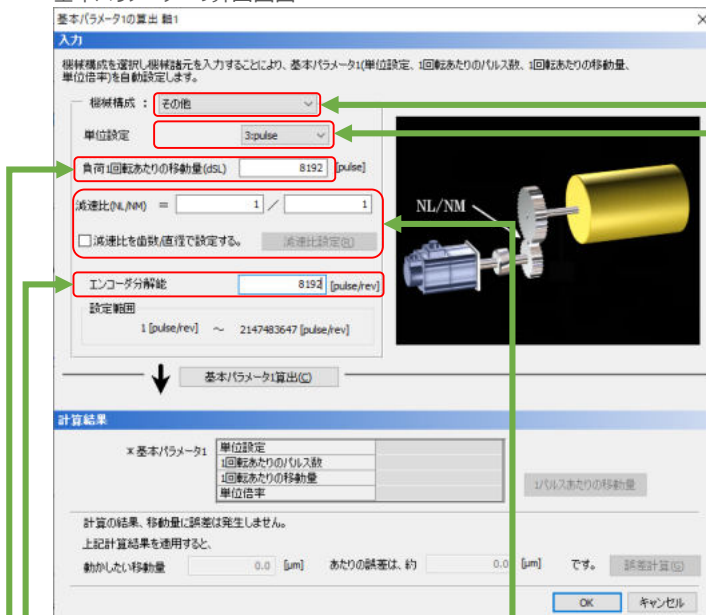
基本パラメータの算出画面
