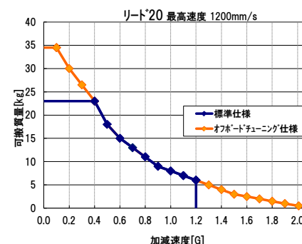
図:加減速度別可搬質量一覧 (ISB-MXM/L 100W) ～水平設置～
