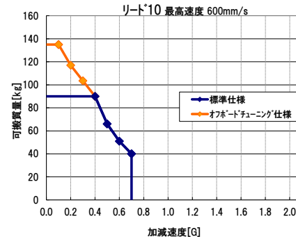
図:加減速度別可搬質量一覧 (ISB-MXM/L 200W) ～水平設置～
