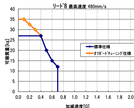
図:加減速度別可搬質量一覧 (ISDBCR-S) ～水平設置～
