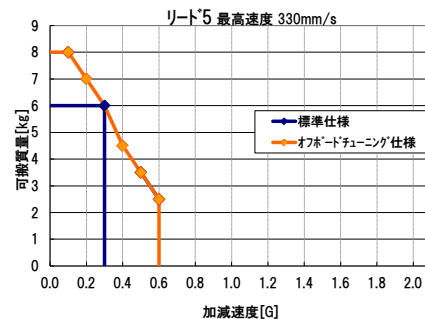
図:加減速度別可搬質量一覧 (RCS2-SA4R) ～水平設置～
