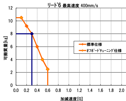
図:加減速度別可搬質量一覧 (RCS2-SA5R) ～水平設置～
