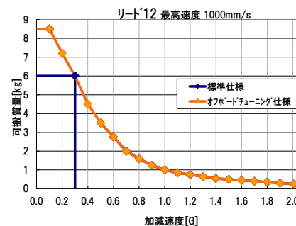
図:加減速度別可搬質量一覧 (RCS2-SA6C) ～水平設置～
