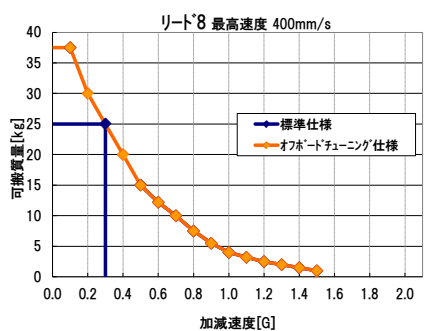
図:加減速度別可搬質量一覧 (RCS2-SA7C) ～水平設置～
