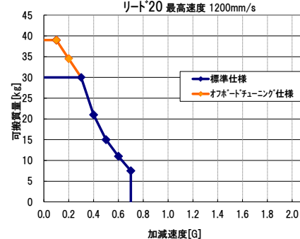
図:加減速度別可搬質量一覧 (RCS3CR-SA8C/SS8C 150W) ～水平設置～
