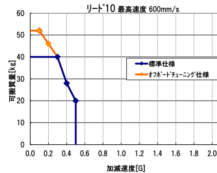
図:加減速度別可搬質量一覧 (RCS3CR-SA8C/SS8C 100W) ～水平設置～
