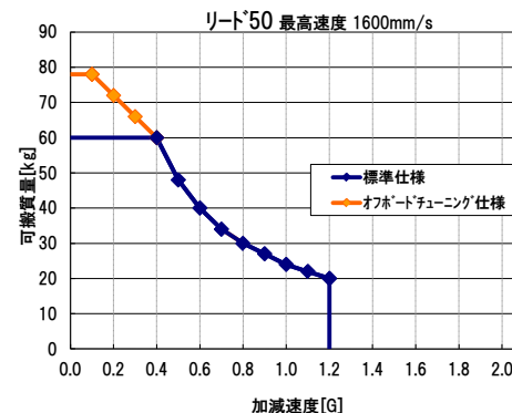
図:加減速度別可搬質量一覧 (SSPDACR-LXM) ～水平設置～
