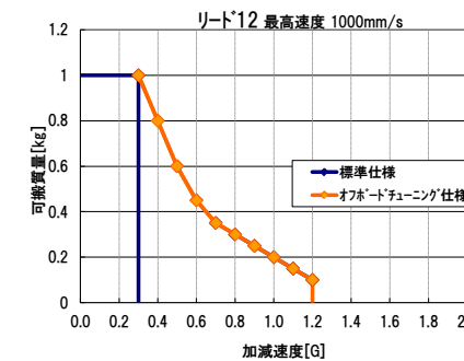
図:加減速度別可搬質量一覧 (RCS2-SA5C) ～垂直設置～
