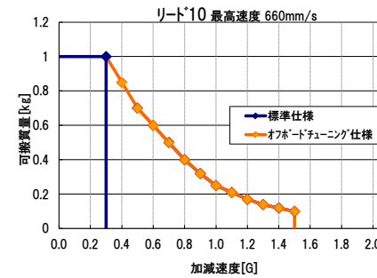
図:加減速度別可搬質量一覧 (RCS2-SA4C) ～垂直設置～
