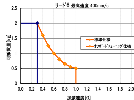
図:加減速度別可搬質量一覧 (RCS2-SA5C) ～垂直設置～
