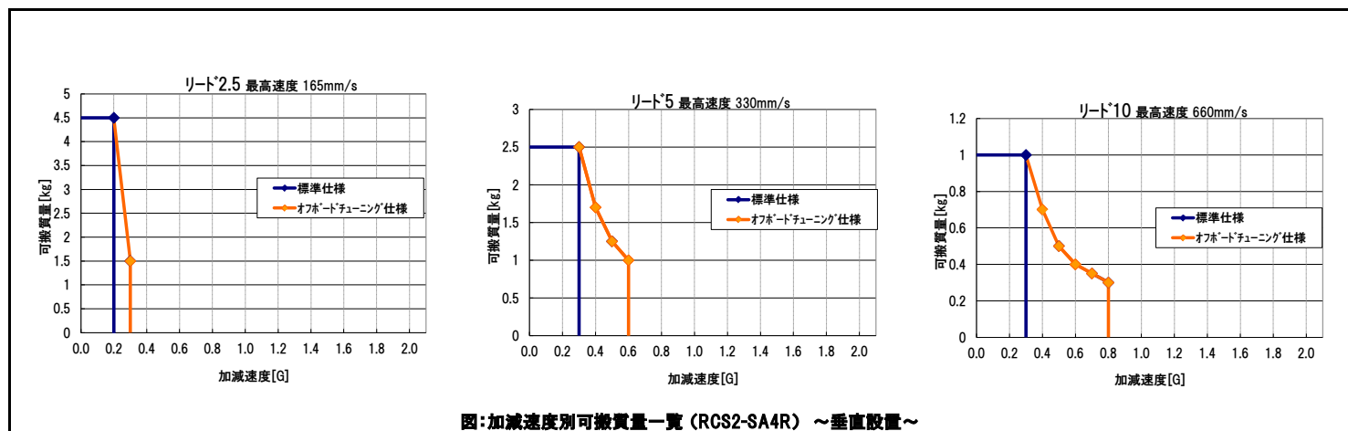
図:加減速度別可搬質量一覧 (RCS2-SA4R) ～垂直設置～
