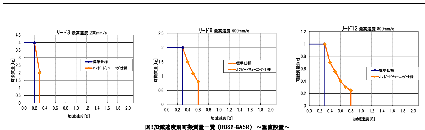
図:加減速度別可搬質量一覧 (RCS2-SA5R) ～垂直設置～
