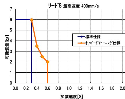
図:加減速度別可搬質量一覧 (RCS2-SA7R) ～垂直設置～
