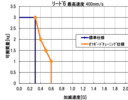
図:加減速度別可搬質量一覧 (RCS2-SA6R) ～垂直設置～
