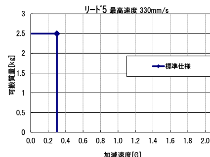
図:加減速度別可搬質量一覧 (RCS2CR-SA4C) ～垂直設置～
