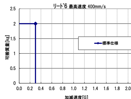
図:加減速度別可搬質量一覧 (RCS2CR-SA5C) ～垂直設置～
