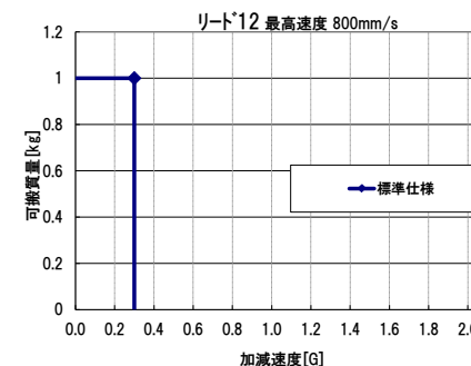
図:加減速度別可搬質量一覧 (RCS2CR-SA5C) ～垂直設置～
